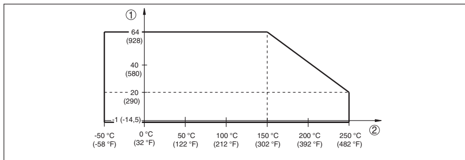
Рис. 17: Температура процесса - давление процесса при установке переключателя \geq 0,5 г/см 3 (переключатель чувствительности)
