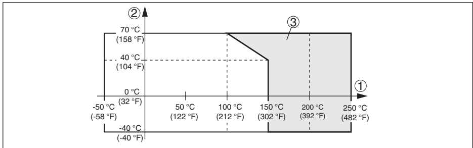
Рис. 15: Температура окружающей среды - Температура процесса
