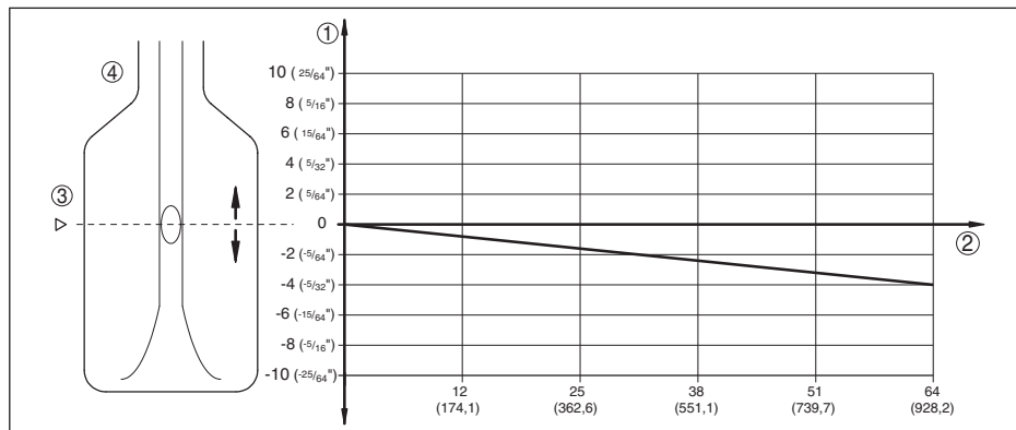
Рис. 14: Влияние давления процесса на точку переключения
