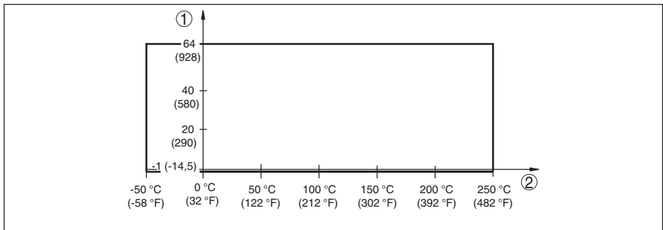
Рис. 16: Температура процесса - давление процесса при установке переключателя \geq 0,7 \text{ г/см}^3 (переключатель чувствительности)
