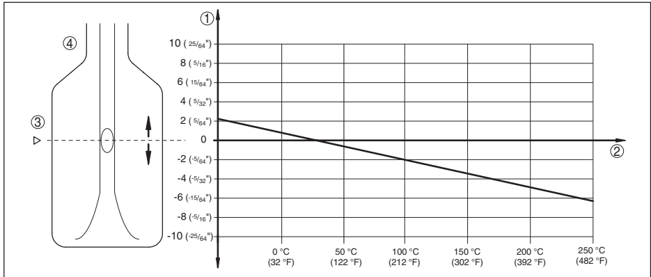
Рис. 12: Влияние температуры процесса на точку переключения
