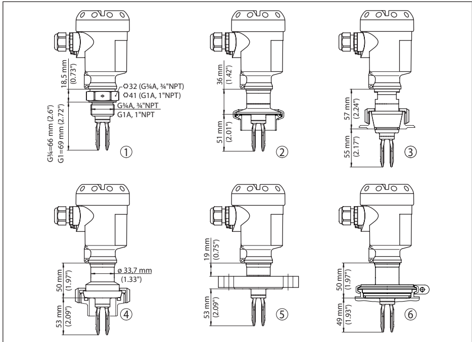
Рис. 19: OPTISWITCH 5100 C, 5150 C
