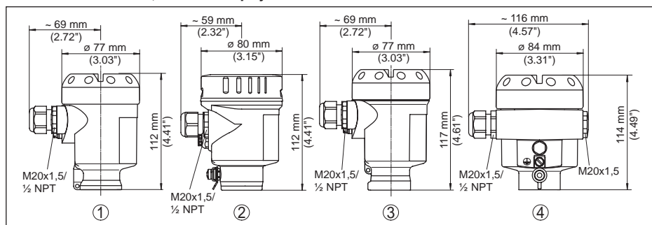
Рис. 18: Исполнения корпуса
