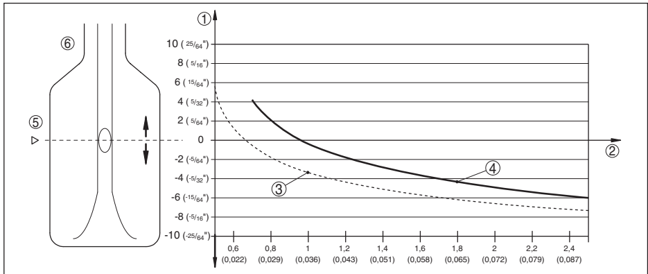
Рис. 13: Влияние плотности продукта на точку переключения
