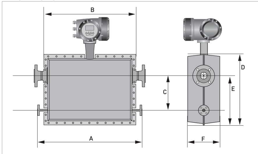
Типоразмеры расходомеров 08...100
