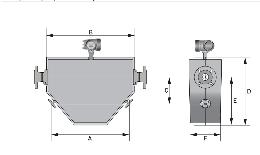
Типоразмеры расходомеров 150...250
