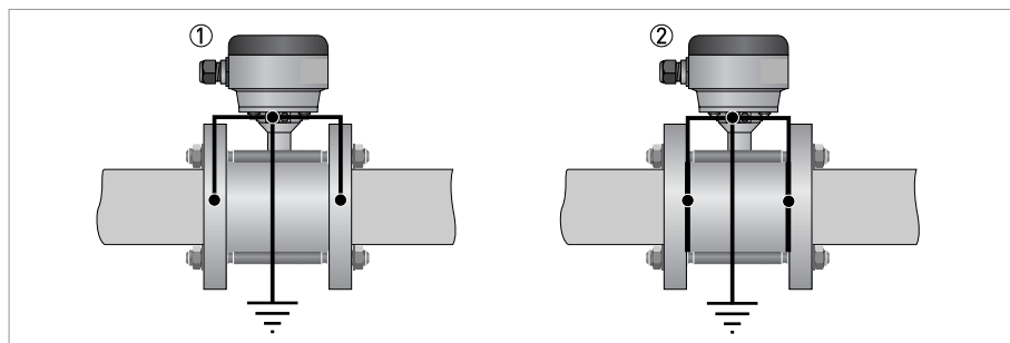
Рисунок 4-1: Заземление
