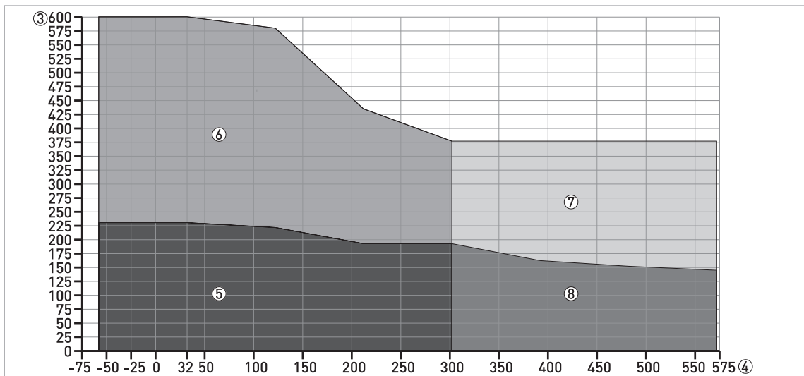
Рисунок 2-6: Номинальное давление / температура (ASME B16.5), фланцевое и резьбовое соединения, в °F и фунт/кв. дюйм изб.
