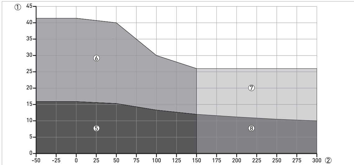
Рисунок 2-5: Номинальное давление / температура (ASME B16.5), фланцевое и резьбовое присоединения, в °C и бар изб.
