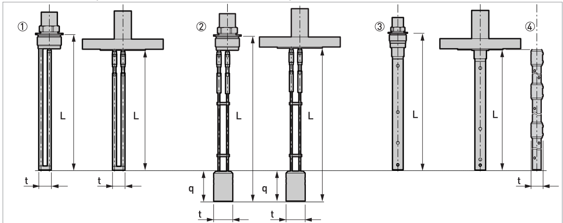
Рисунок 2-14: Варианты сдвоенных стержневых и коаксиальных сенсоров
