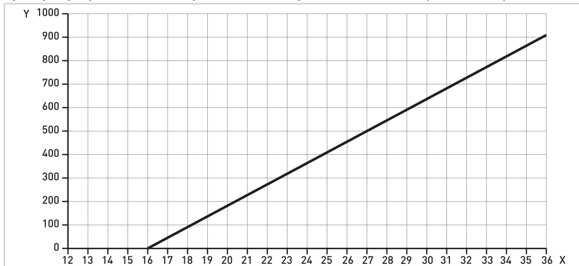
Рисунок 2-2: Минимальное напряжение источника питания при выходном токе 22 мА на клеммах прибора (исполнение для работы во взрывоопасных зонах (Ex d / XP/NI))
