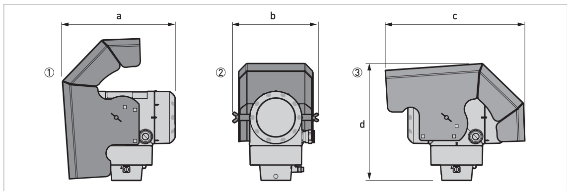
Рисунок 2-12: Опция защиты от погодных условий для компактной / горизонтальной версии и раздельной версии
