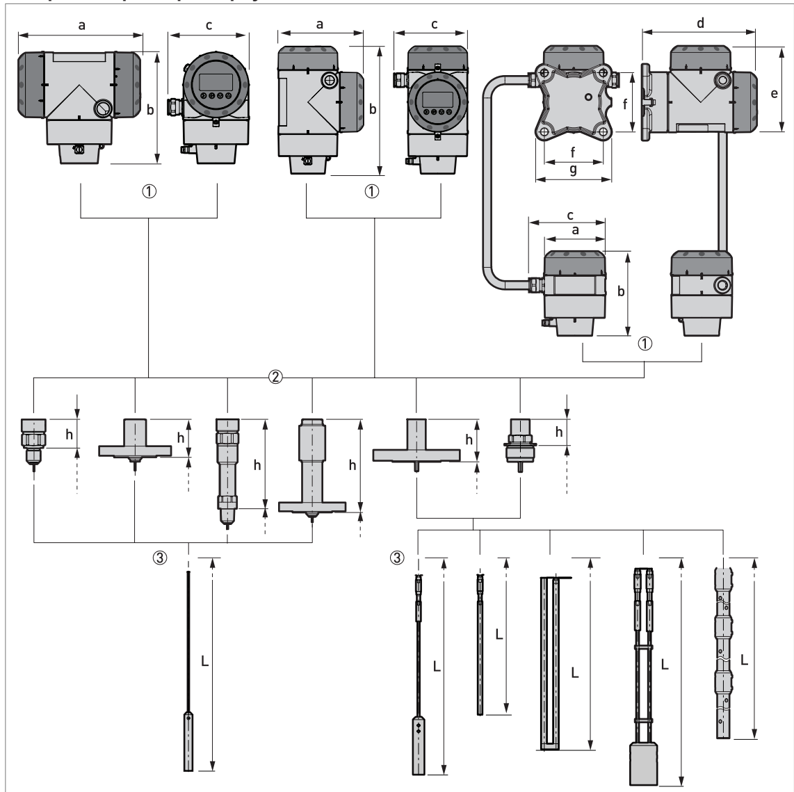
Рисунок 2-10: Габаритные размеры корпуса
