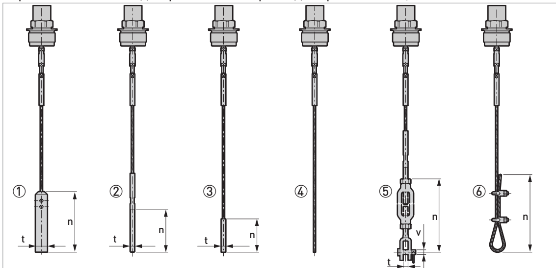
Рисунок 2-15: Варианты окончаний одностросовых сенсоров: один трос \varnothing 4 \text{ мм}/0,15''
