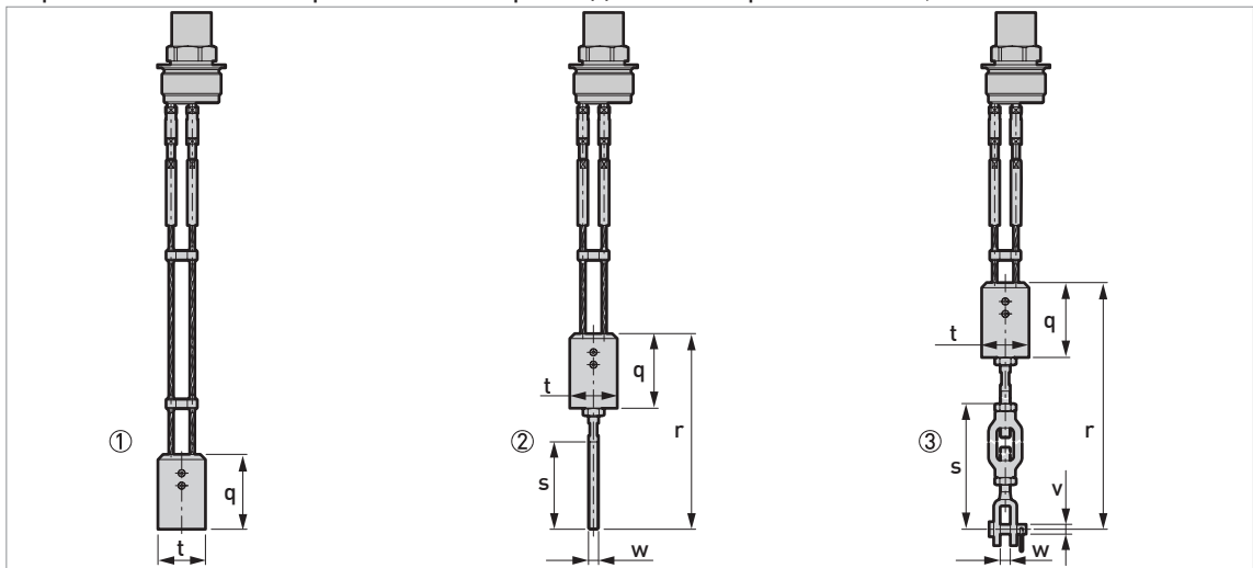
Рисунок 2-16: Варианты окончаний тросовых сенсоров: сдвоенный трос \varnothing 4 \text{ мм}/0,15''
