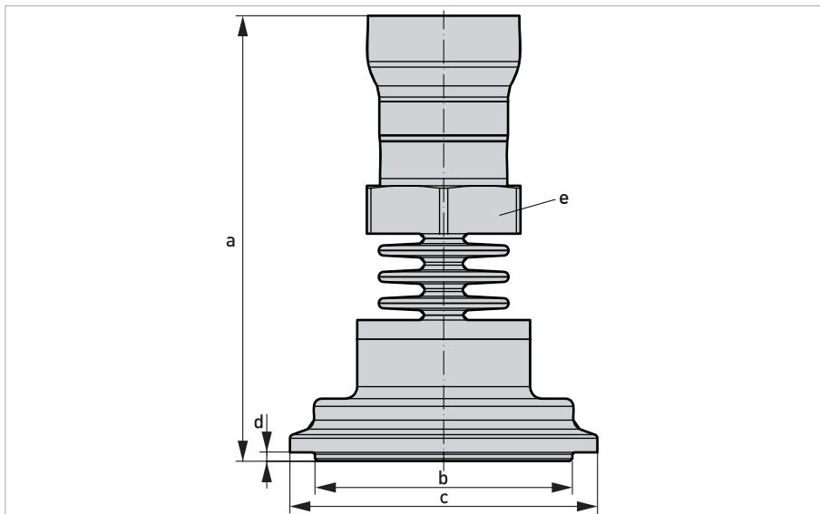
Рисунок 2-13: Асептическое зажимное соединение DIN 11864-3 форма А
