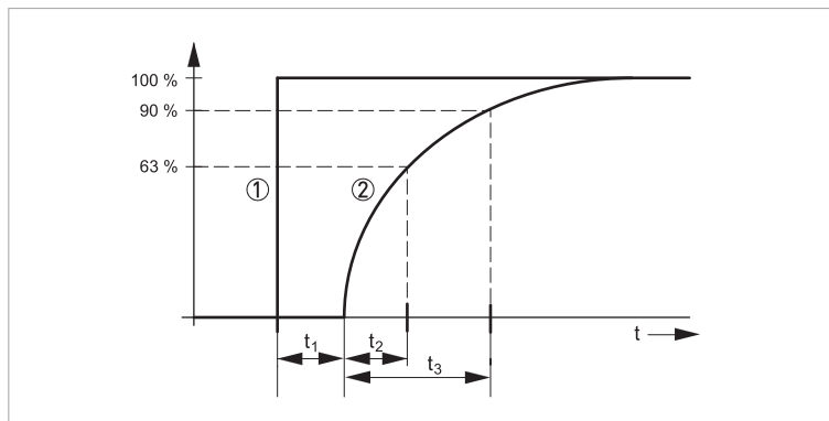
Рисунок 2-18: Характеристика при резком изменении технологического параметра. t_1 - время запаздывания; t_2 - время нарастания t_{63} ; t_3 - время нарастания t_{90}
